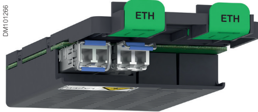
Ethernet HSR/PRP FO module
